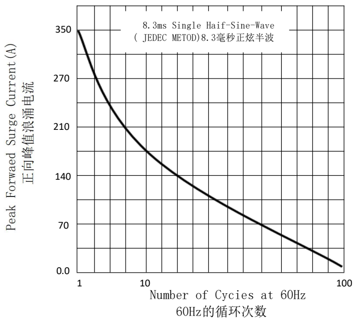
图2 最大不重复正向浪涌曲线
