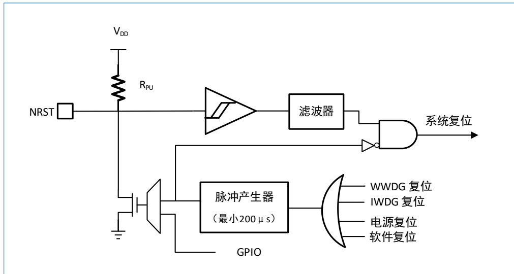
图 3-3 复位电路
