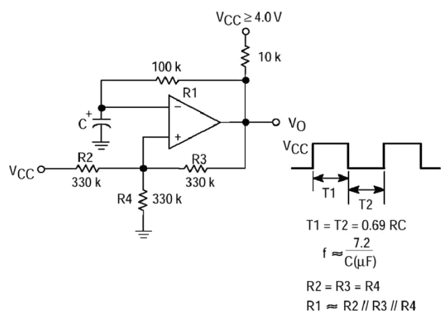
方波振荡器
