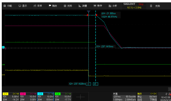
UVLO protection
