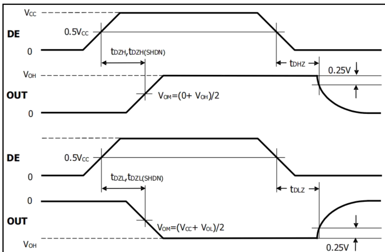
图 6.驱动器使能和禁用时序( t_{DHZ} 、 t_{DZH} 、 t_{DZH}(SHDN) 、 t_{DZL} 、 t_{DLZ} 、 t_{DLZ}(SHDN) )
