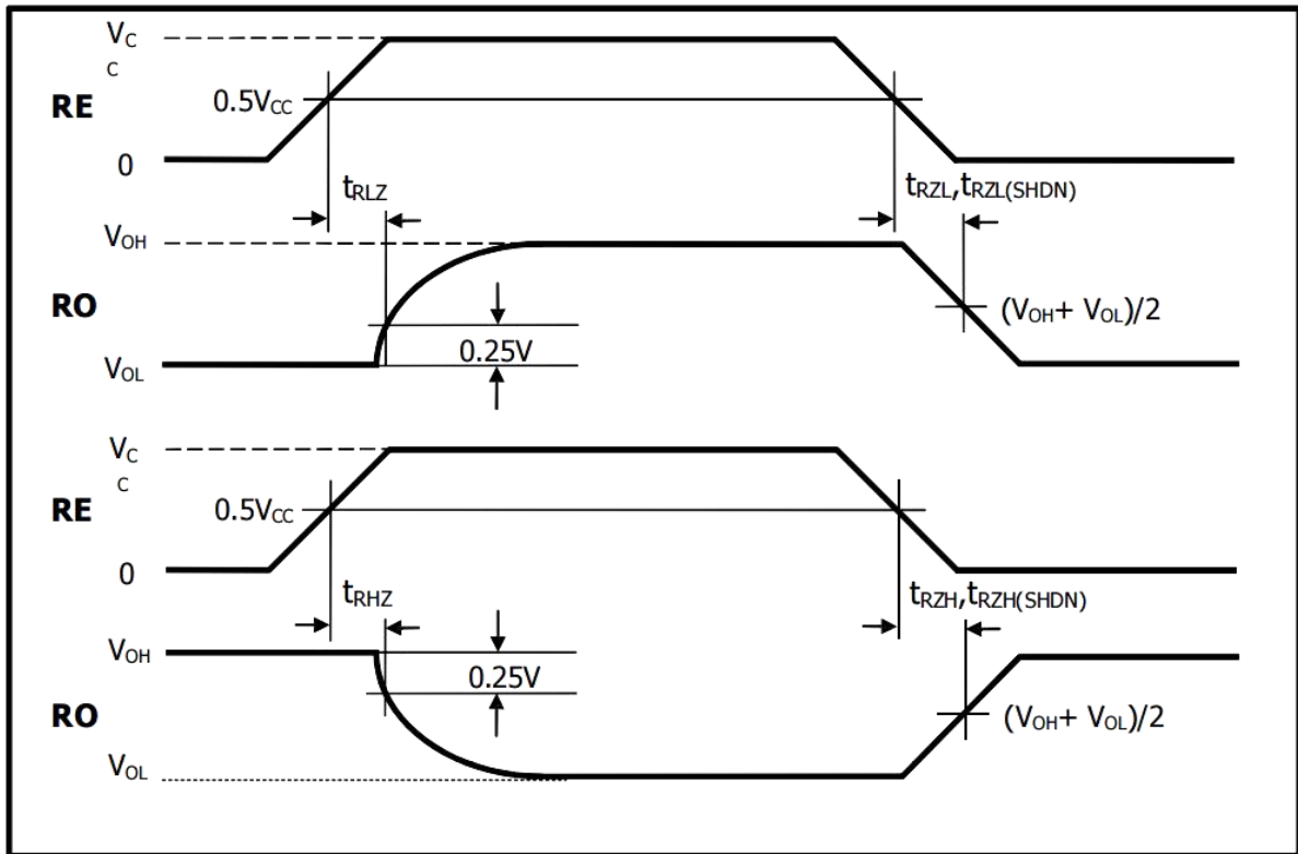
图 9.接收器使能和禁用时序
