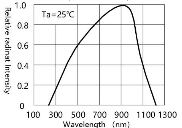
感应波长曲线图 Spectral Sensitivity
