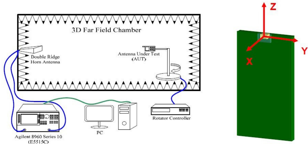
Fig.2 暗室示意图 FAR-field Chamber
