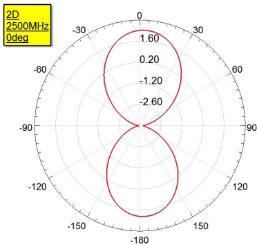
2D 增益模式 2D Gain Pattern (2500 MHz)
