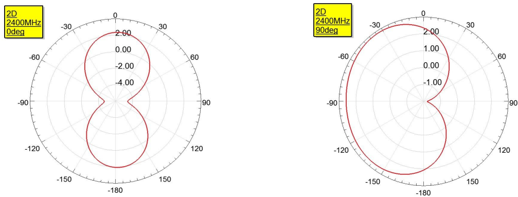
2D 增益模式 2D Gain Pattern (2400 MHz)
