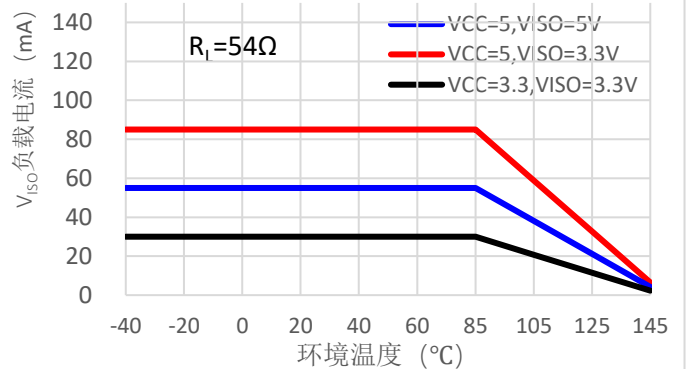
图 7.10-18 V_{ISO} 最大负载可用电流随器件环境温度的变化 A 和 B 之间 R_L=54\Omega TDA51S485HC: DR=500kbps, A 和 B 之间 C_L=2nF
