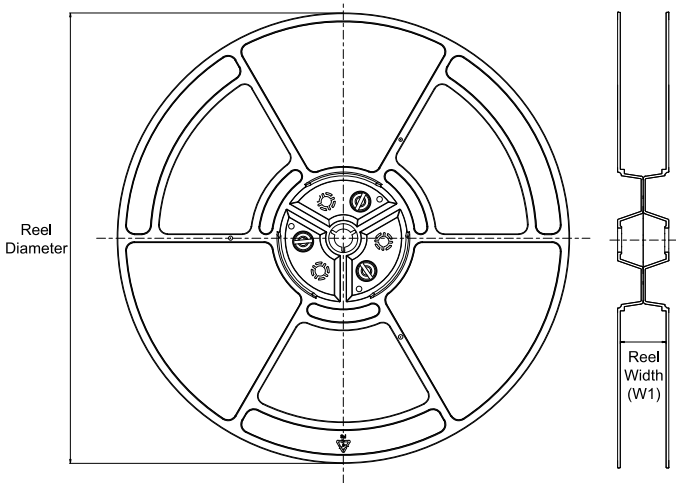
REEL DIMENSIONS
