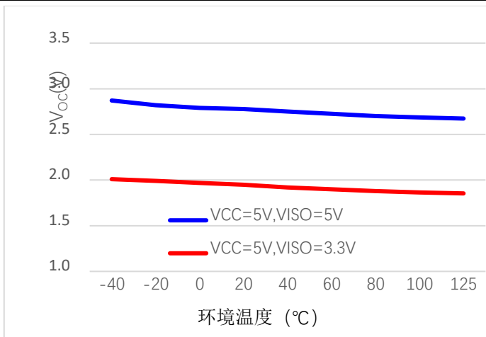
图 7.10-12 共模输出电压 V_{OC} , R_L = 54\Omega , V_{CC} = 5\text{V}
