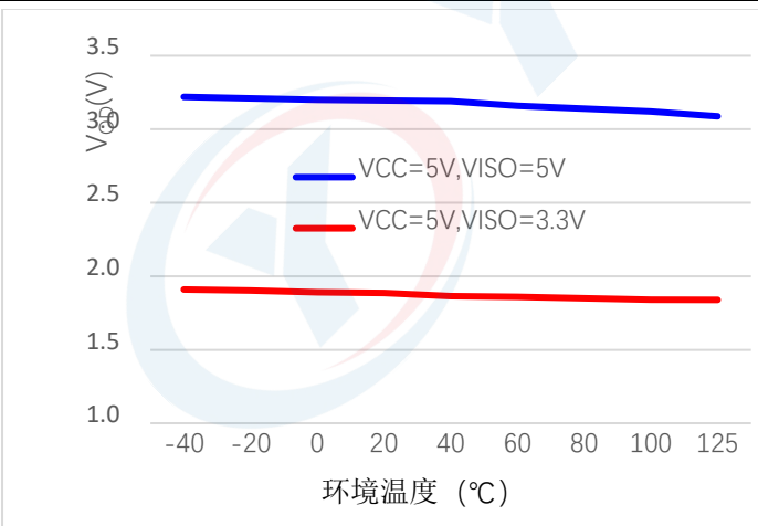
图 7.10-11 差模输出电压 V_{OD} , R_L = 54\Omega , V_{CC} = 5\text{V}
