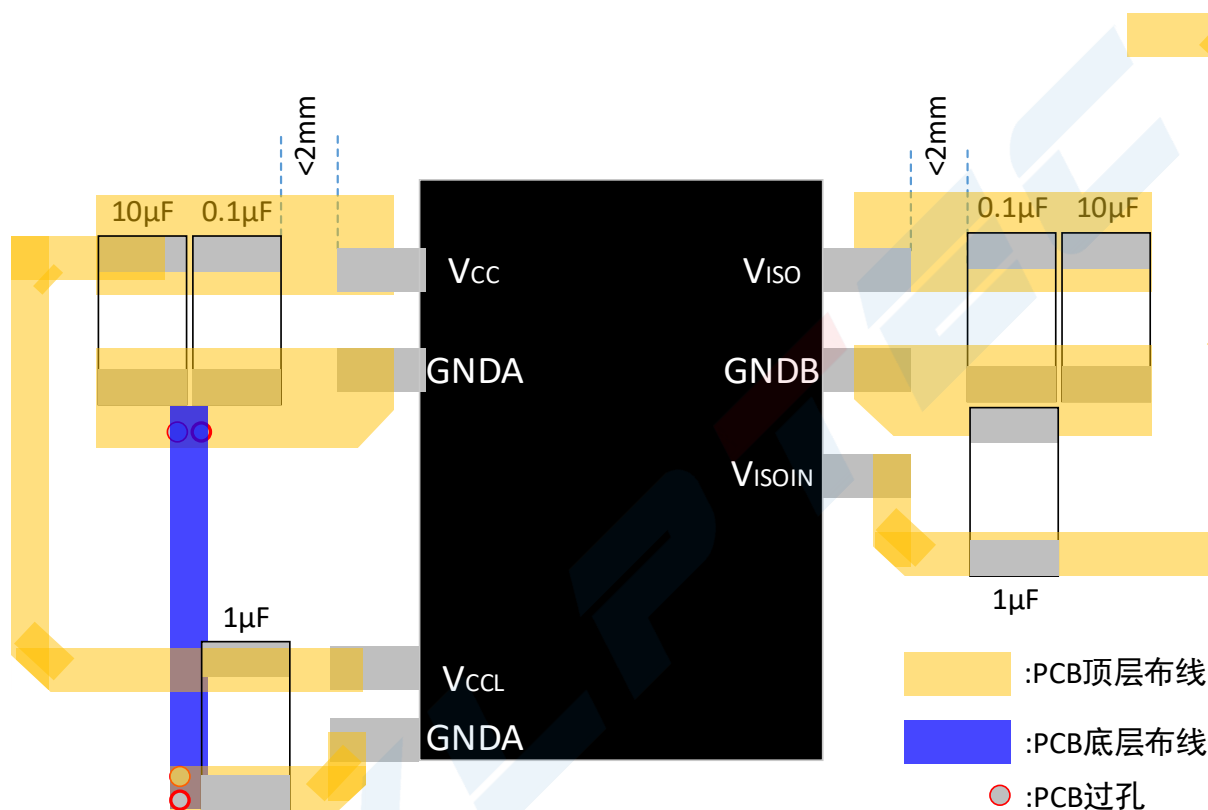
图 10-3 推荐 PCB 电源部分走线
