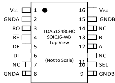
图 6-1 TDA51S485HC引脚分布
