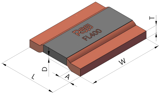
标准图尺寸
