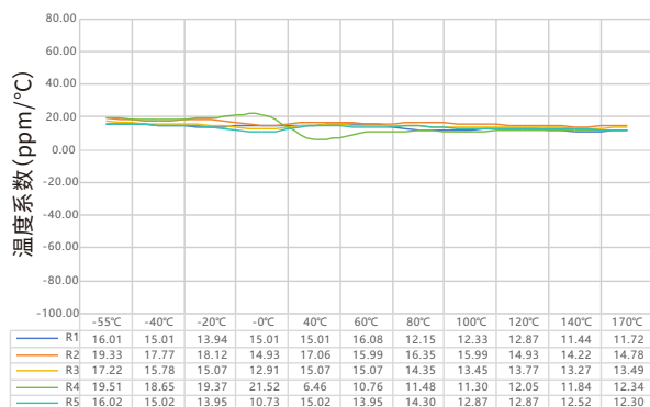
SEWK3951系列0.25mΩ温度系数实测数据表
