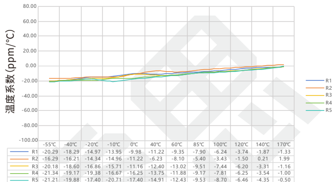
SEWK3951系列0.4mΩ温度系数实测数据表
