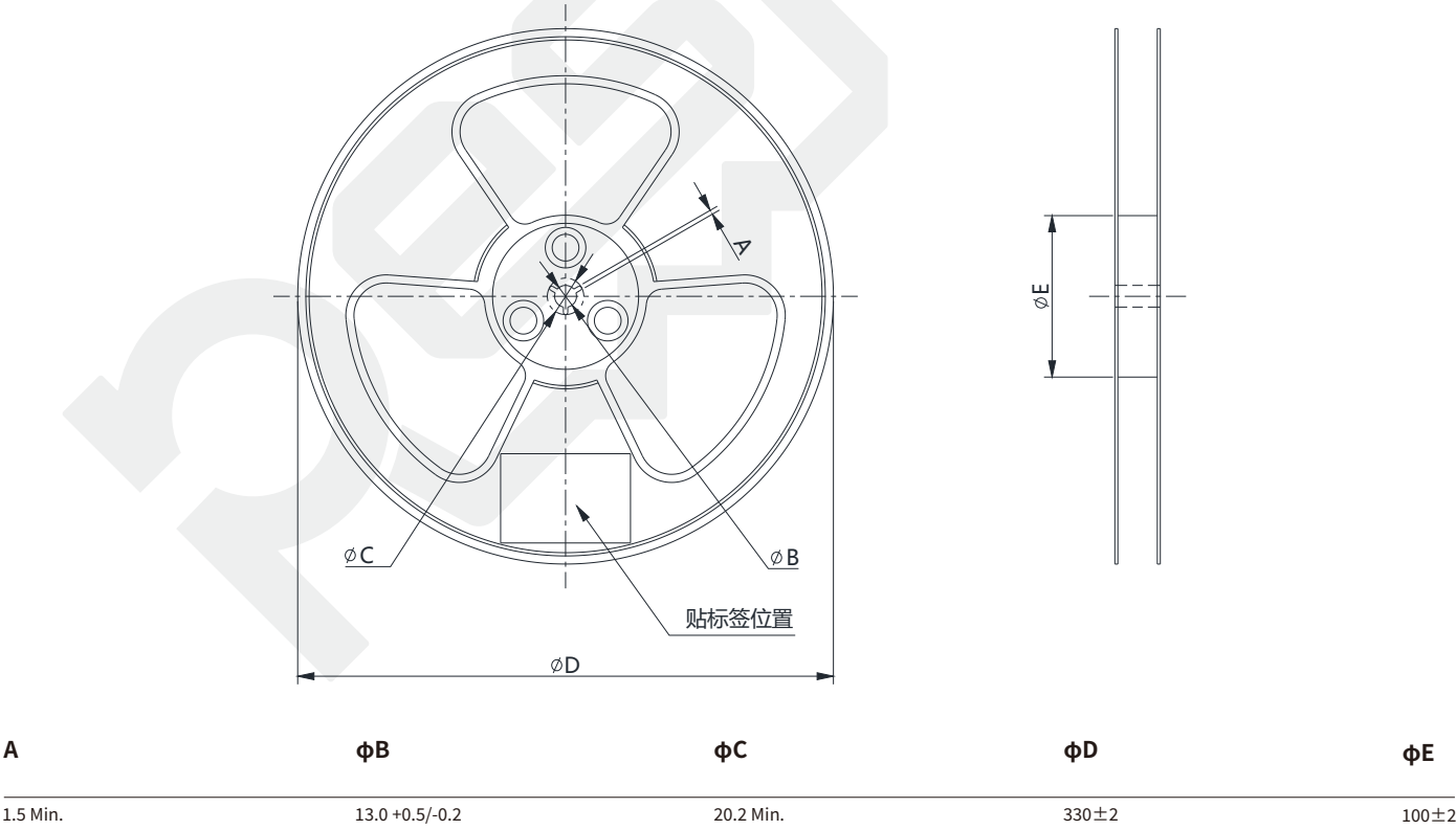
卡盘尺寸图
