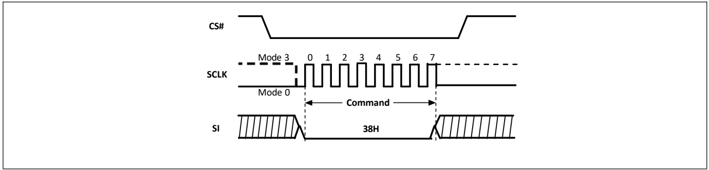
Figure-67. Enable QPI (QPI)
