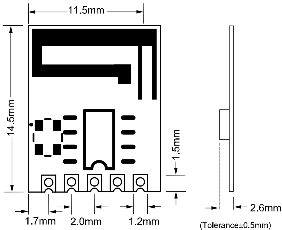
图 3-1：模组尺寸
