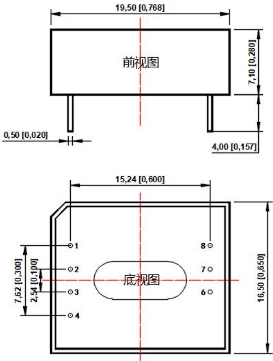
外观尺寸图
