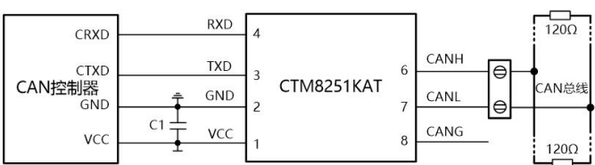
CAN 控制器 3.3V 供电应用电路（图 2）
