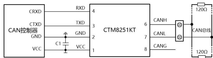
CAN 控制器 5V 供电应用电路（图 1）
