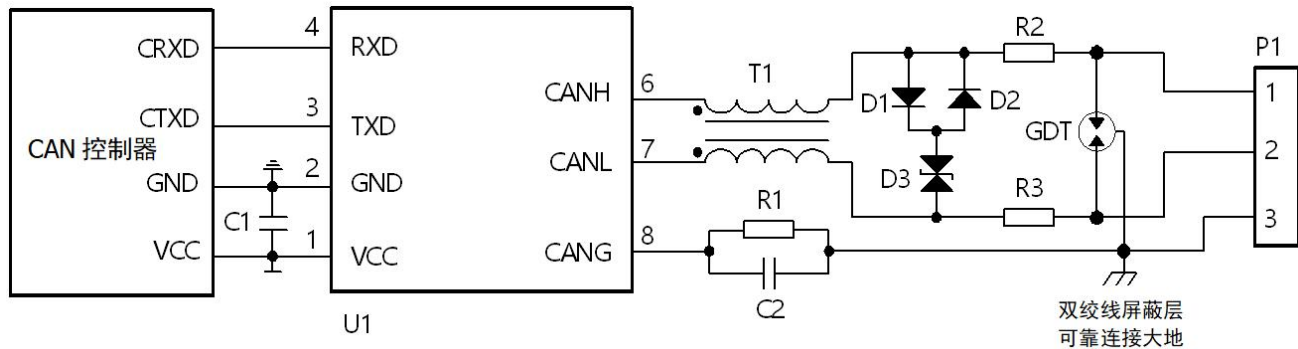
EMC 推荐电路（图 4）
