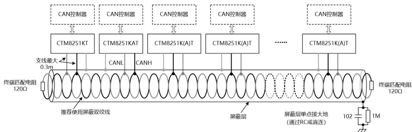
单个 CAN-Bus 典型网络连接示意图（图 3）
