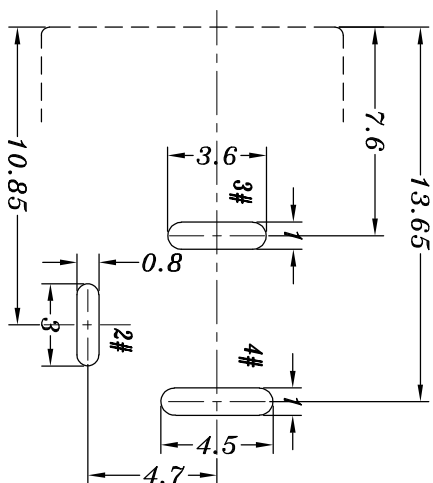
P.C.B LAYOUT
