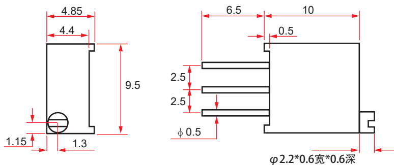
结构及尺寸 (mm) Dimensions and Structure(mm)
