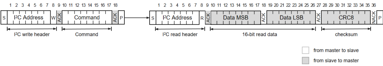
图 5 GXHTV4 的典型 I 2 C 通信时序
