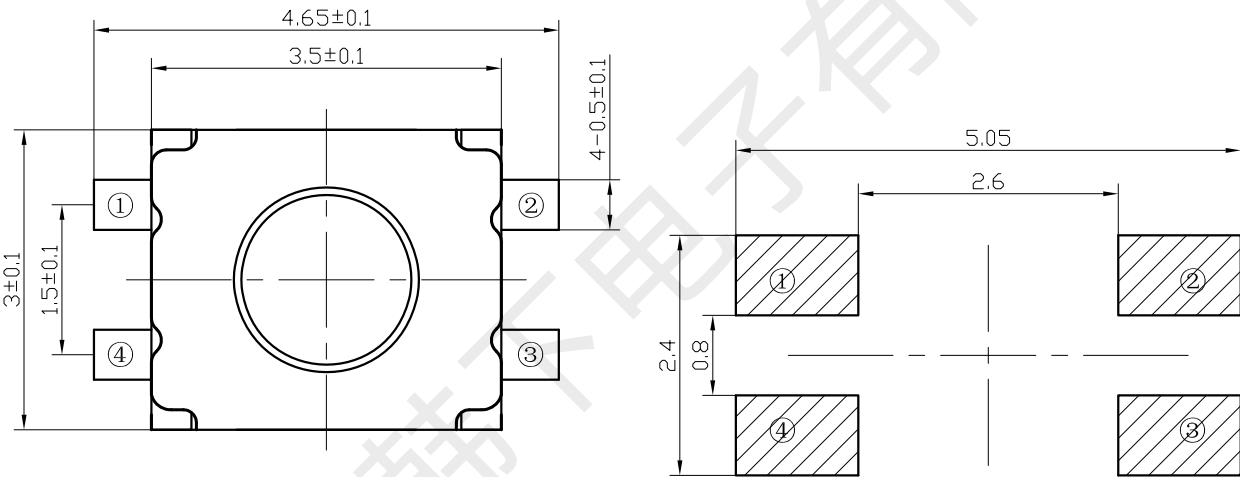
安装参考图
