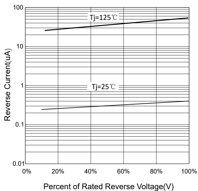
FIG 3: V_R - I_R
