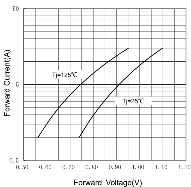
FIG 4: I_F - V_F
