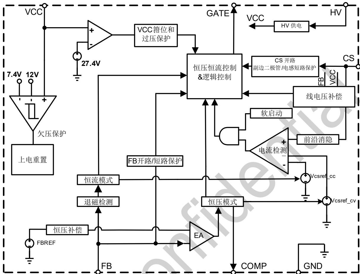
图 3. BP3529B 内部框图
