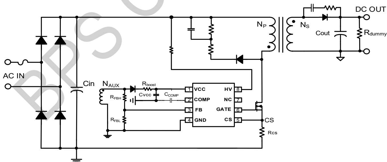
图 1. BP3529B 典型应用电路
