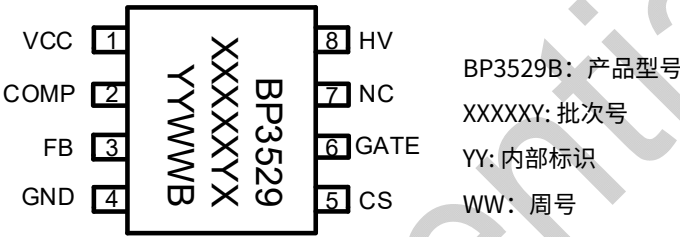
图 2. SOP-8 管脚封装图
