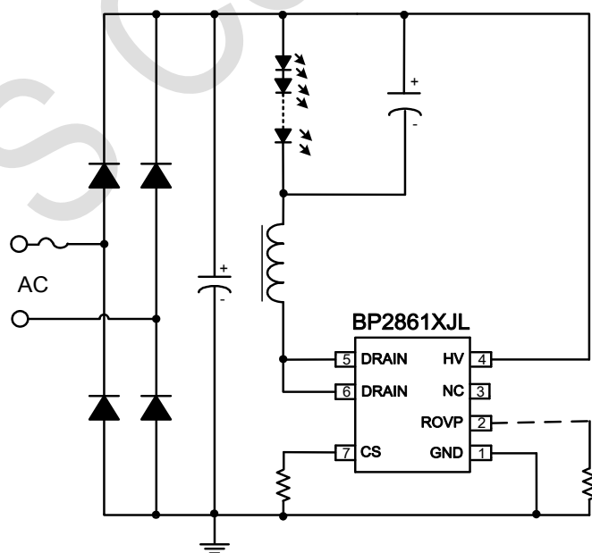
图 1 BP2861XJL 典型应用图
