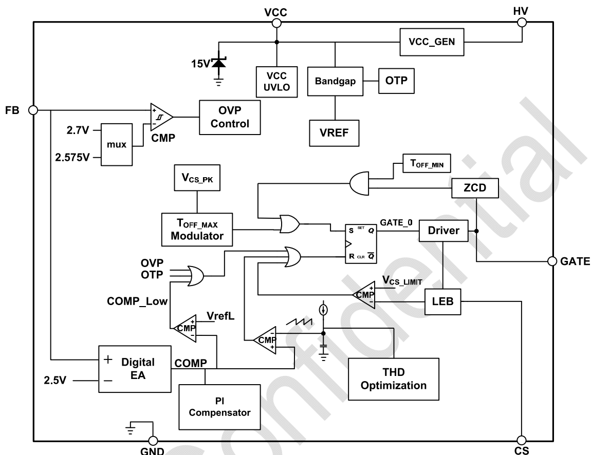
图 3 BP2639A 内部框图
