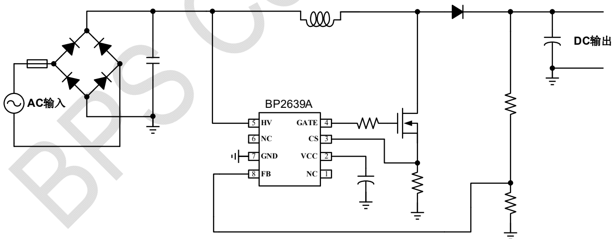
图 1 BP2639A 典型应用电路
