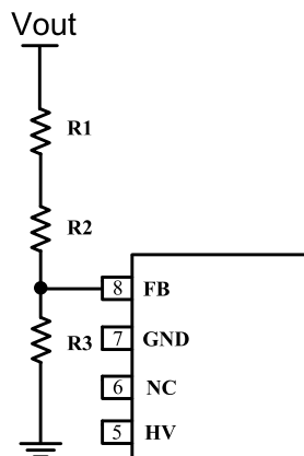
图 4 FB 引脚应用示意图
