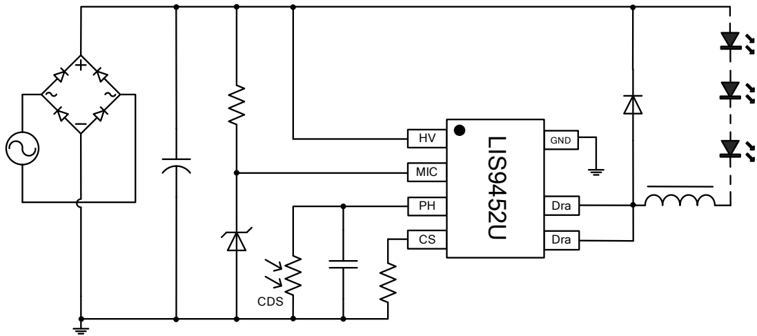
图2 典型纯光控应用电路
