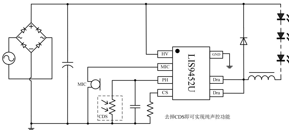
图1 典型声光控或纯声控应用电路
