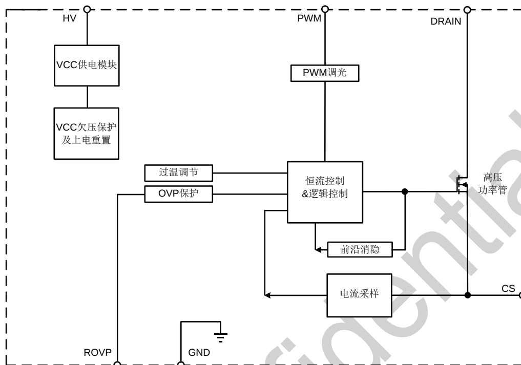
图 3 BP2956XH 内部框图
