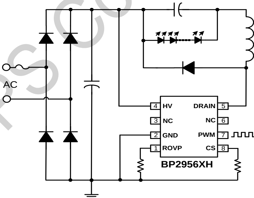
图 1 BP2956XH 典型应用图
