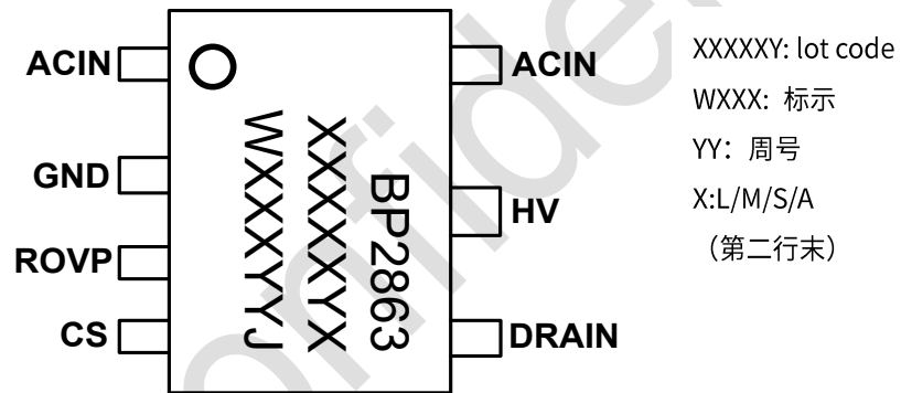
图 2 管脚封装图
