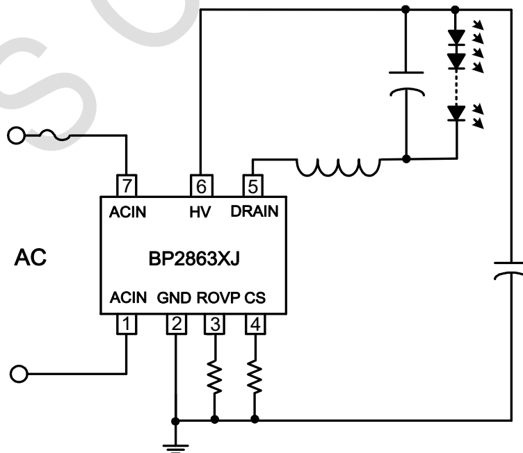
图 1 BP2863XJ 典型应用图
