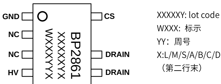
图2 管脚封装图
