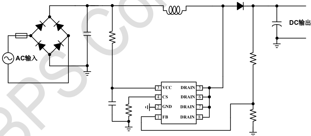
图 1 BP2636CA 典型应用电路
