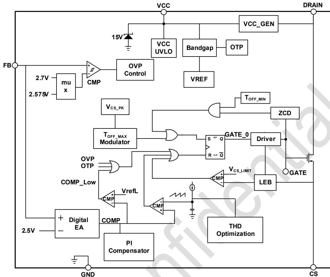
图 3 BP2636CA 内部框图
