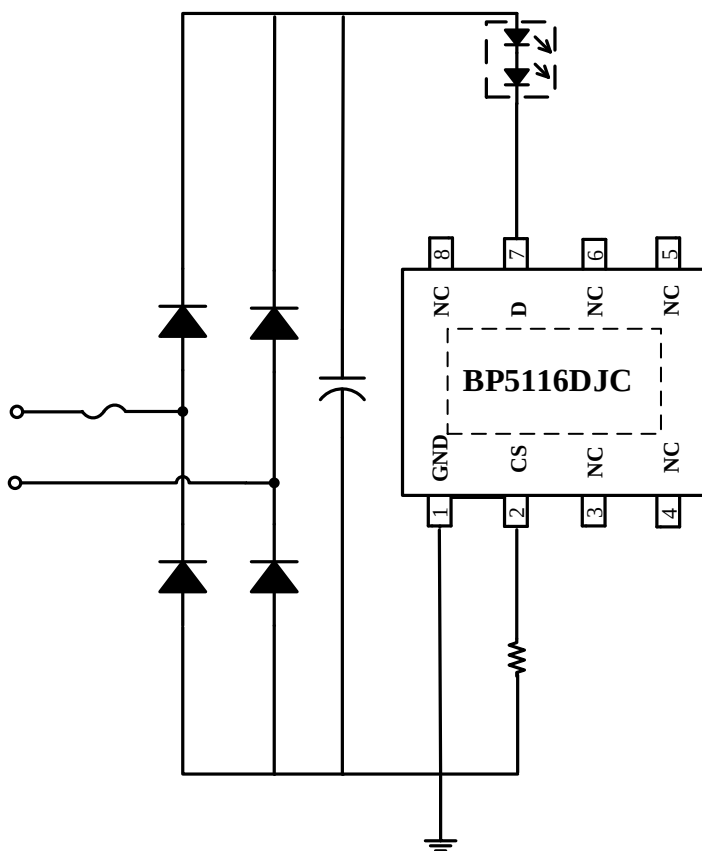
图 1 BP5116DJC 典型应用图
