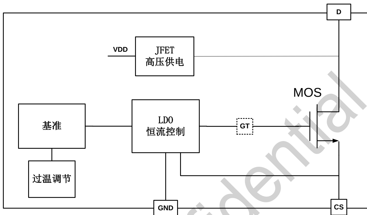
图 3 BP5116DJC 内部框图
