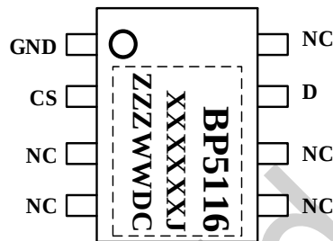
图 2 BP5116DJC 管脚封装图
