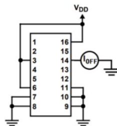
Fig.2 相邻通道关闭漏电流
