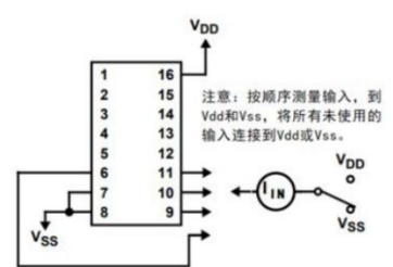
Fig.4 输入电流
