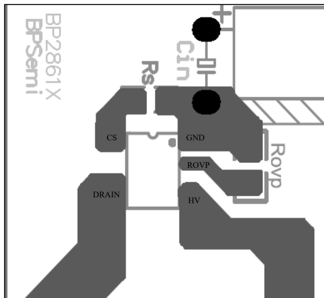
图 4 PCB 铺铜面积优化图
