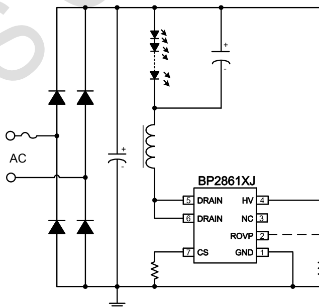
图 1 BP2861XJ 典型应用图
