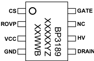
图 2 管脚封装图
