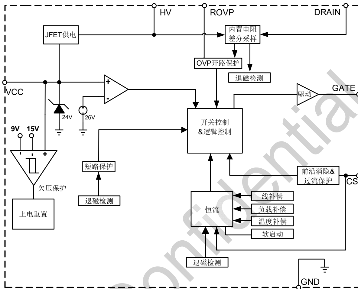
图 3 BP3189B 内部框图
