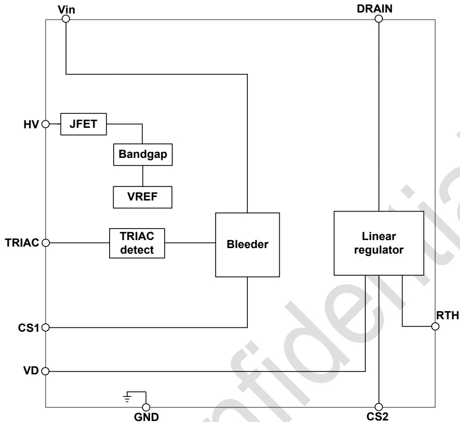
图 3 BP5188GCL 内部框图
