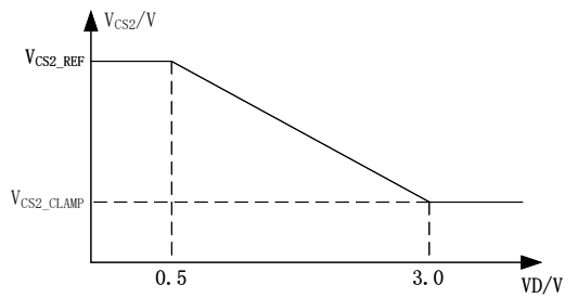
图 4 VD 线补偿曲线
