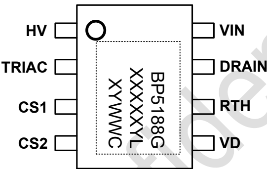
图 2 管脚封装图
