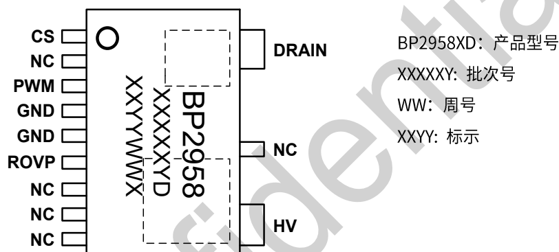
图 2 管脚封装图
