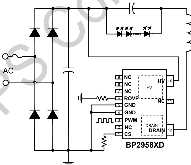
图 1 BP2958XD 典型应用图
