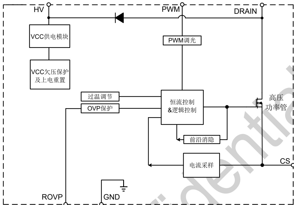
图 3 BP2958XD 内部框图
