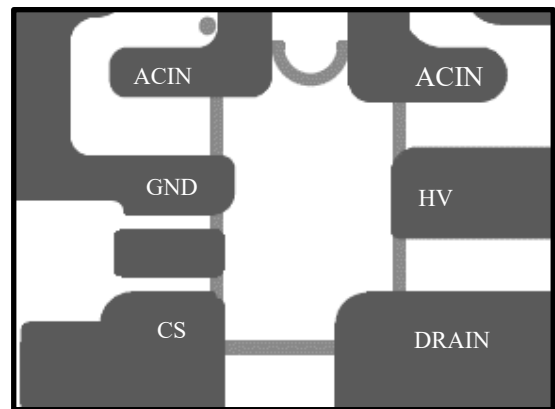
图 4 PCB 铺铜面积优化图
