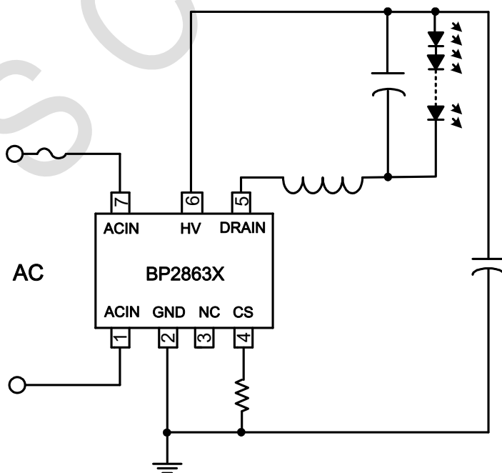
图 1 BP2863X 典型应用图
