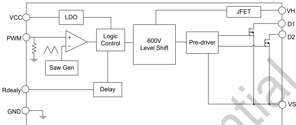
图 3. BP5826D 内部框图
