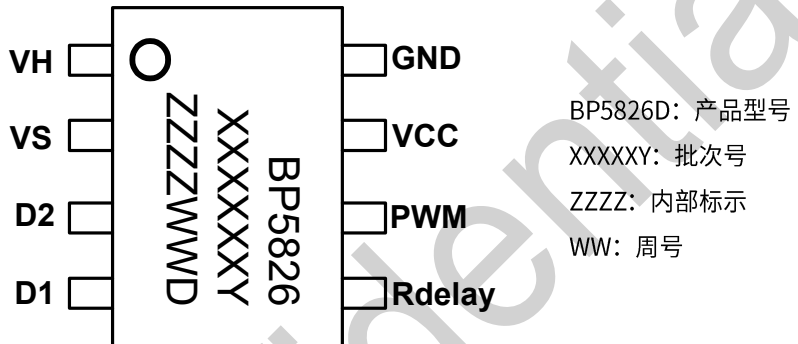
图 2. 管脚封装图
