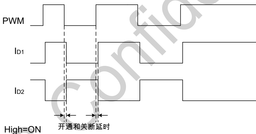
图 4. PWM 调色时序图
