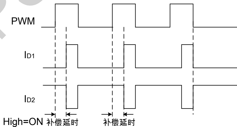
图 5. 色温补偿时序图
