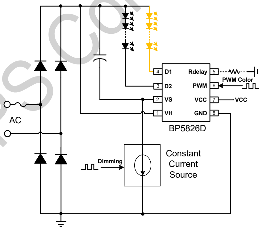
图 1. BP5826D 典型应用图
