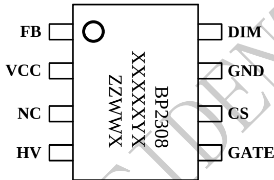
图 2 管脚封装图
