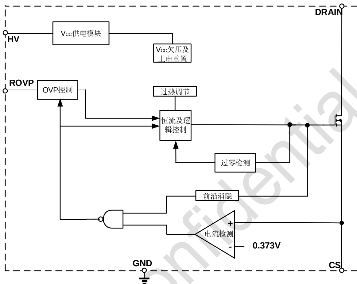
图 3 BP2867FJN 内部框图
