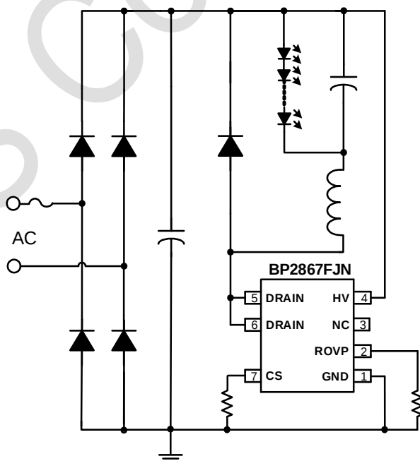
图 1 BP2867FJN 典型应用图
