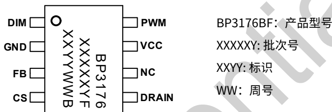
图 2. 管脚封装图
