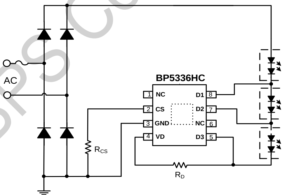
图 1 BP5336HC 典型应用图
