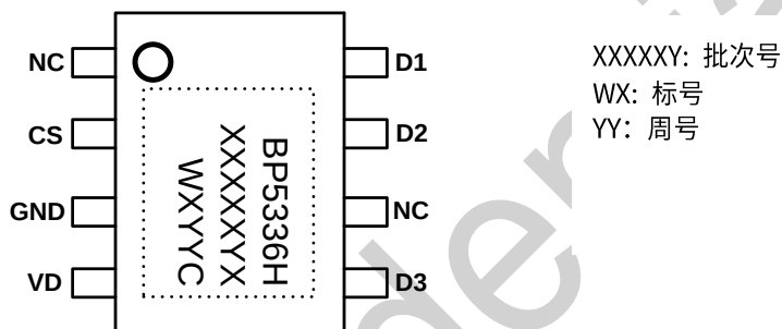
图 2 管脚封装图
