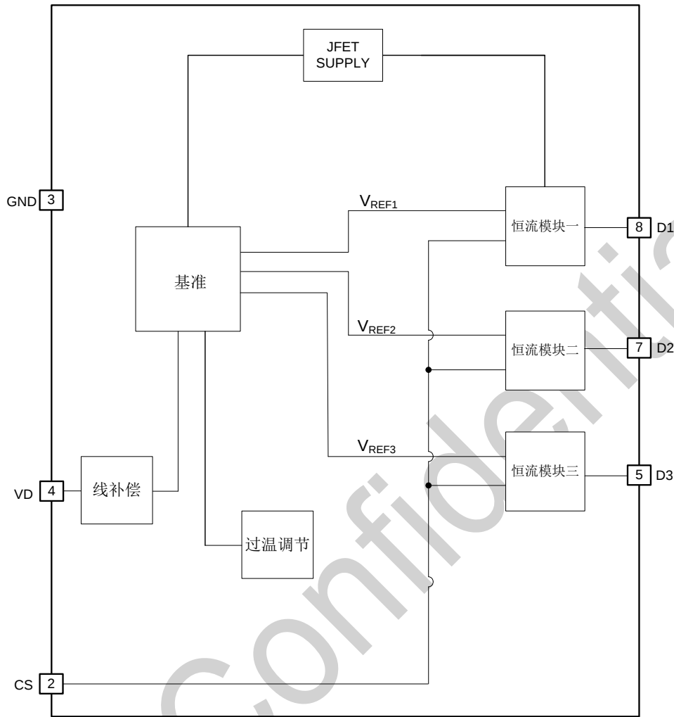
图 3 BP5336HC 内部框图
