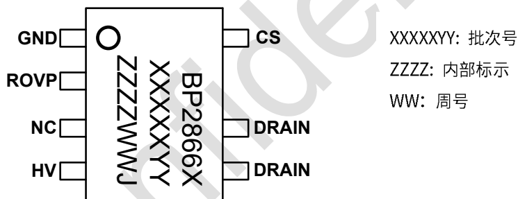
图 2 管脚封装图
