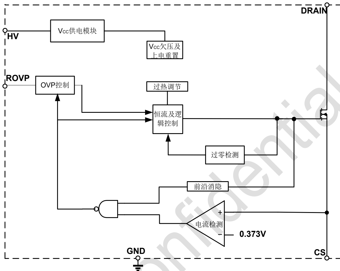
图 3 BP2866XJ 内部框图
