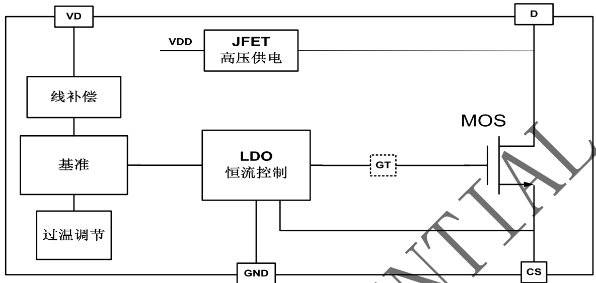
图 3 BP5151DK 内部框图
