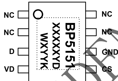
图 2 BP5151DK 管脚封装图
