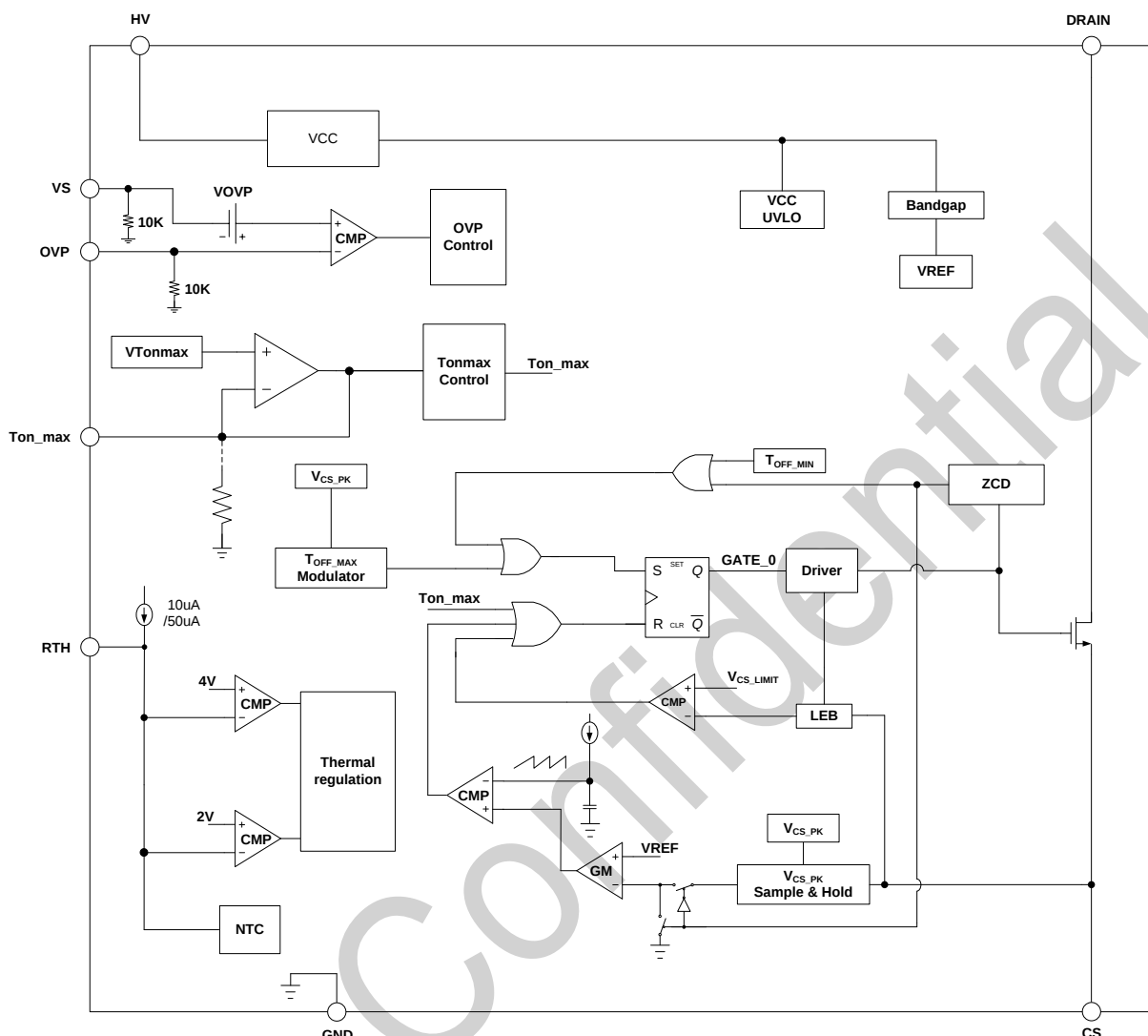
图 3. BP3286CLN 内部框图
