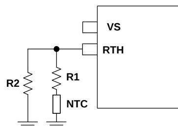
图 6. NTC 参考线路
