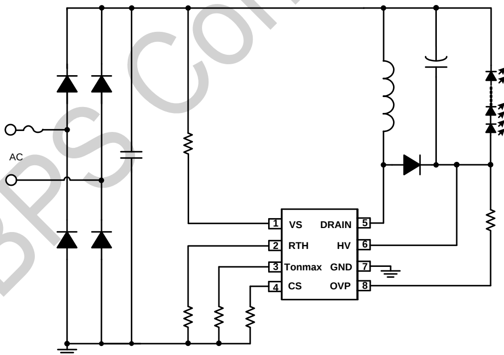
图 1. BP3286CLN 典型应用图 (Buck-Boost)
