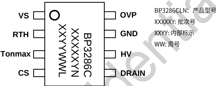
图 2. SOP-8 管脚封装图
