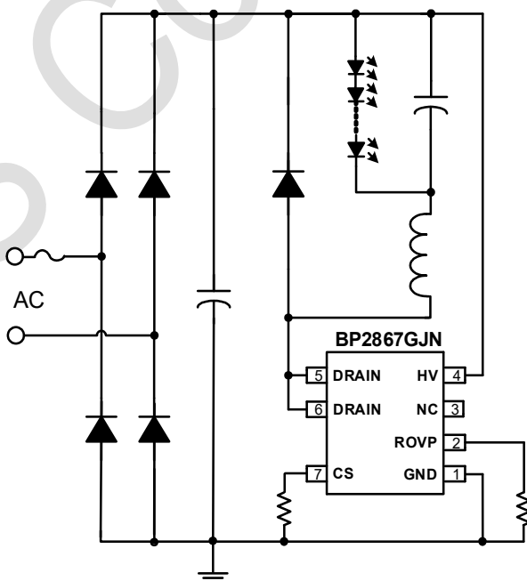
图 1 BP2867GJN 典型应用图
