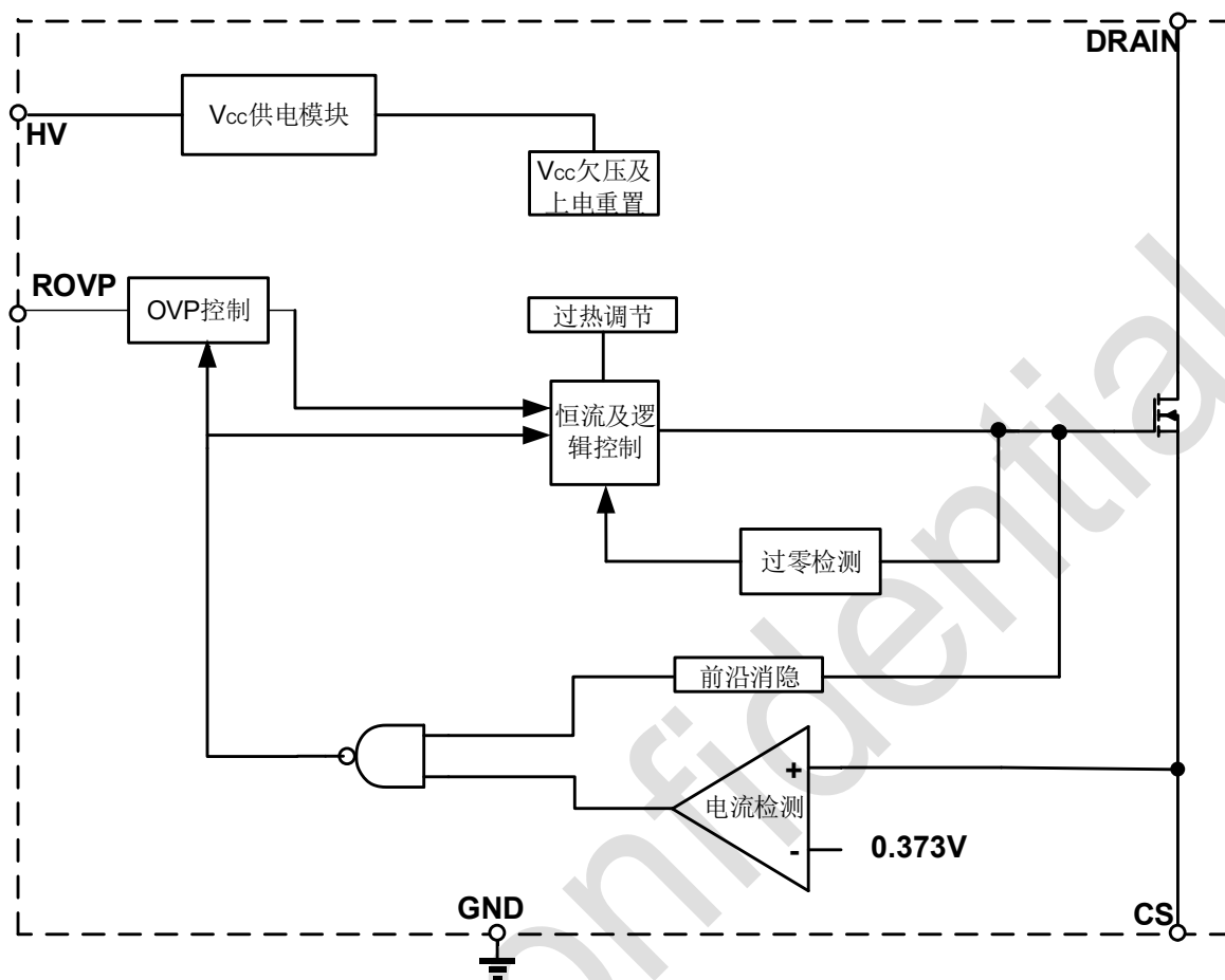
图 3 BP2867GJN 内部框图
