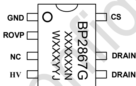
图 2 管脚封装图
