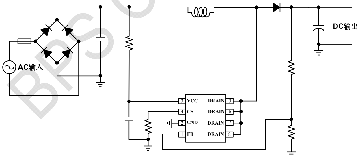
图 1 BP2636CL 典型应用电路
