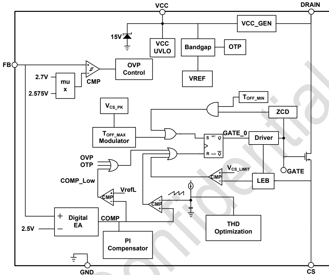
图 3 BP2636CL 内部框图
