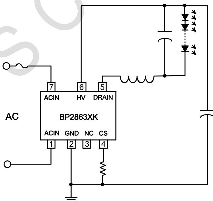
图 1 BP2863XK 典型应用图
