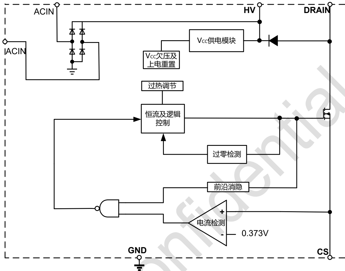
图 3 BP2863XK 内部框图
