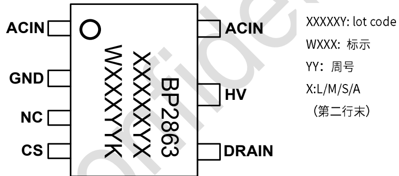
图 2 管脚封装图
