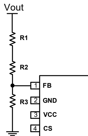
图 4 FB 引脚应用示意图
