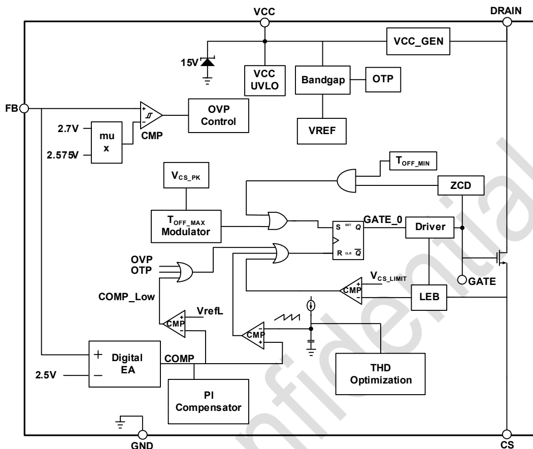
图 3 BP2636DA 内部框图
