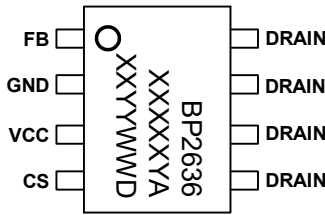
图 2 SOP-8 管脚封装图
