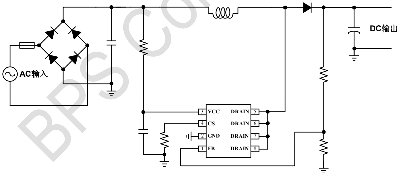
图 1 BP2636DA 典型应用电路
