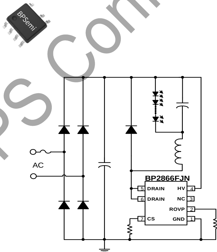
图 1 BP2866FJN 典型应用图
