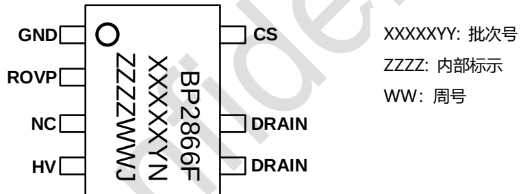
图 2 管脚封装图
