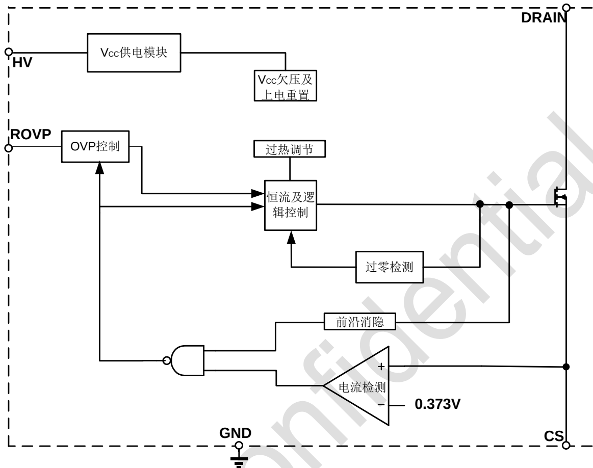
图 3 BP2866FJN 内部框图
