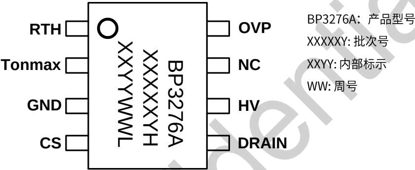
图 2. SOP-8 管脚封装图
