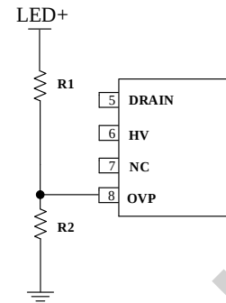
图 5. OVP 线路示意图
