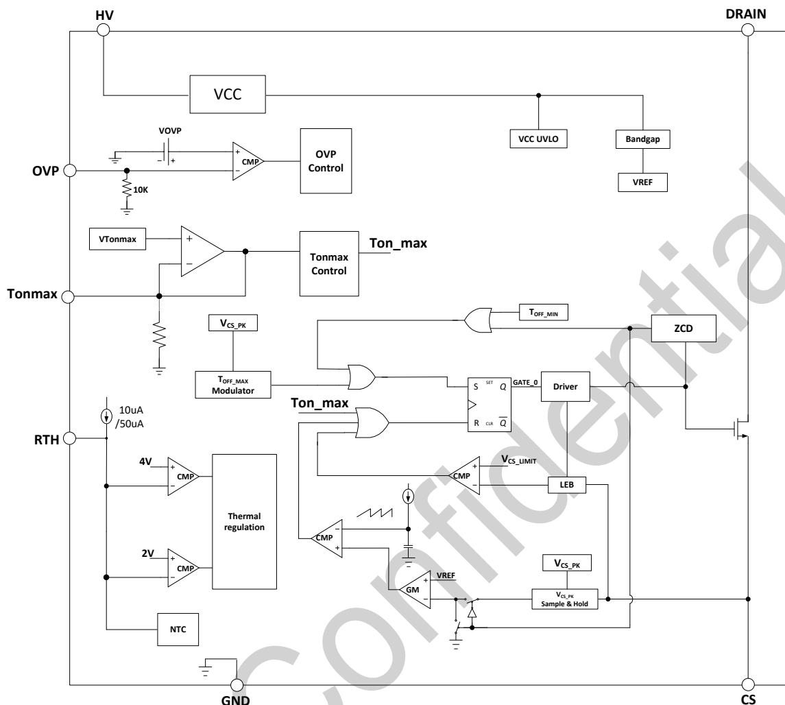
图 3. BP3276AHL 内部框图
