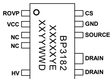
图 2 管脚封装图
