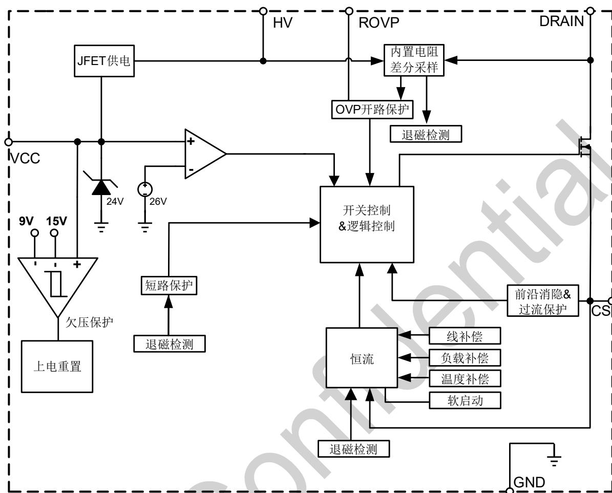
图 3 BP3182ED 内部框图
