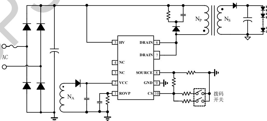
图 1 BP3182ED 典型应用电路
