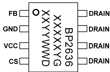
图 2.SOP-8 管脚封装图
