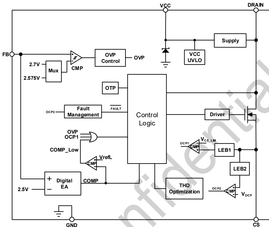
图 3. BP2636DG 内部框图
