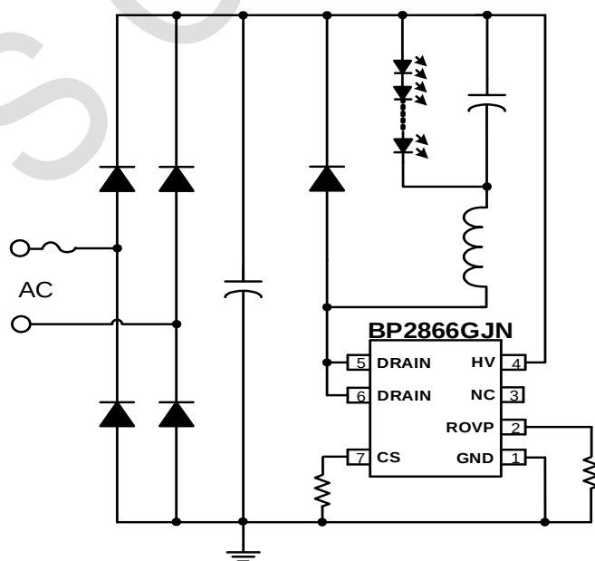
图 1 BP2866GJN 典型应用图
