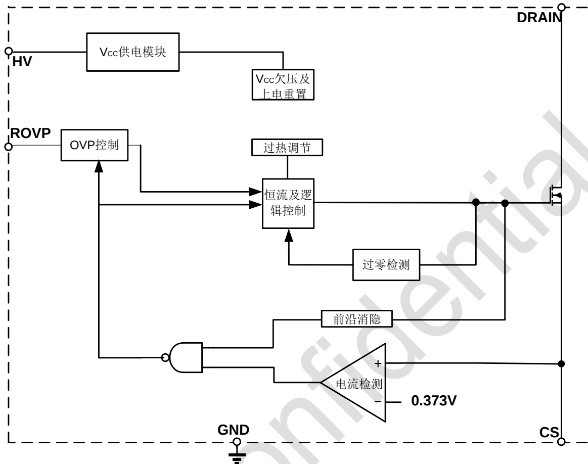
图 3 BP2866GJN 内部框图
